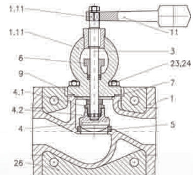
Ventil für Zinnschmelze, mit Heizmantel und Schnellabsperung globe valve for tin melt, with heating case and immediate closure stem
